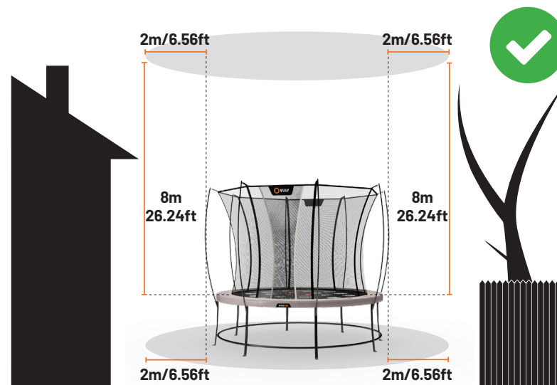
Korrekte Installation
